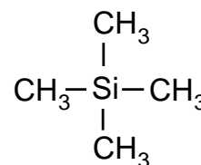
TETRAMETHYLSILANE
